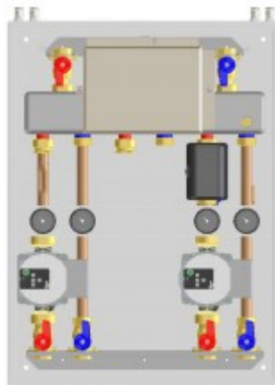
MODUŁ WIELOSTRELOWY - SIM WP 2Z typ CZUJNIK TEMPERATURY ZEWNĘTRZNEJ 1LTE.1HT.YP
